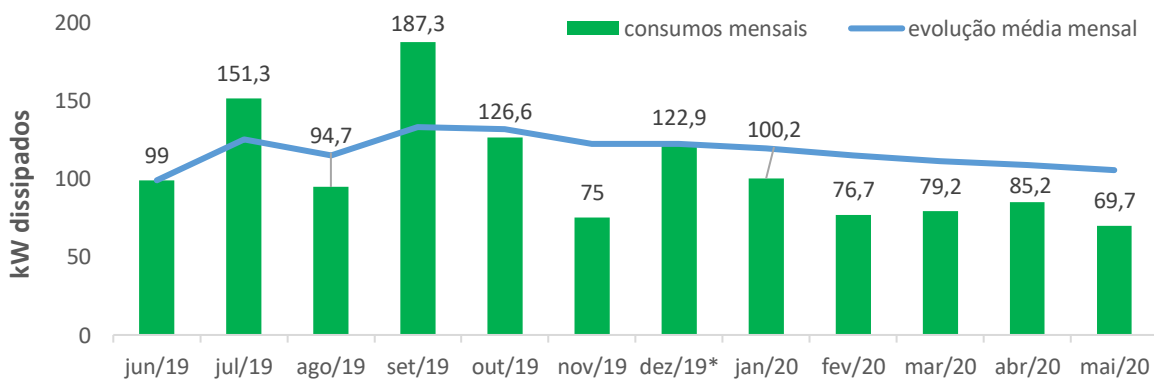
Figura 3 - Evolução da potência elétrica dissipada pelos clusters:
