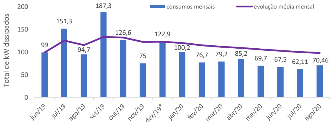
Figura 3 - Evolução da potência elétrica dissipada em kW:
