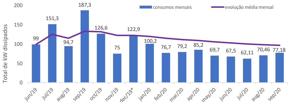
Figura 3 - Evolução da potência elétrica dissipada em kW:
